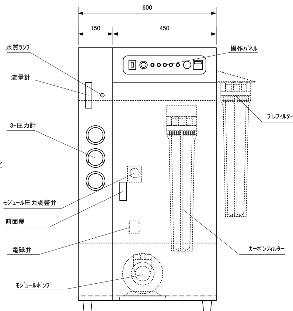
【正面】
