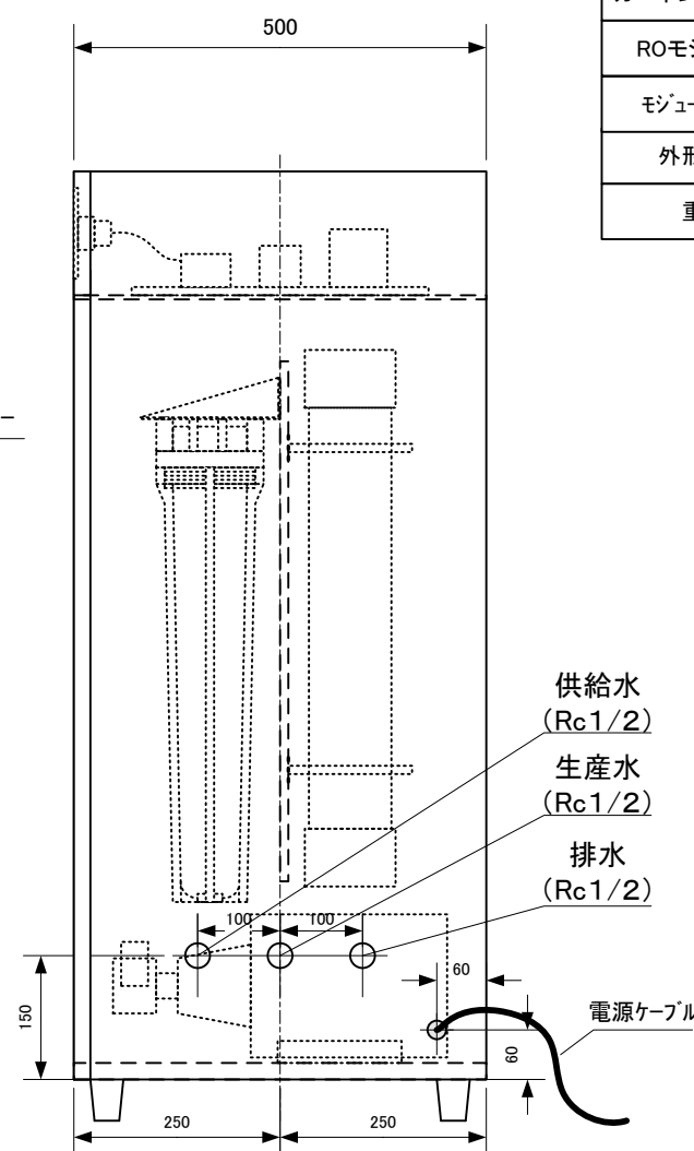
【右側面】
