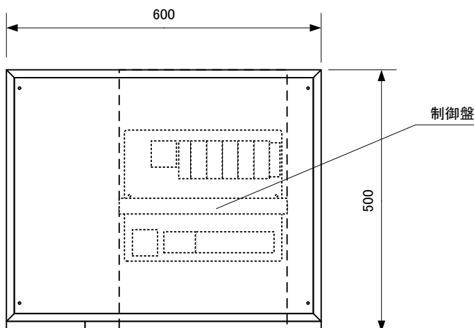
【上面】
