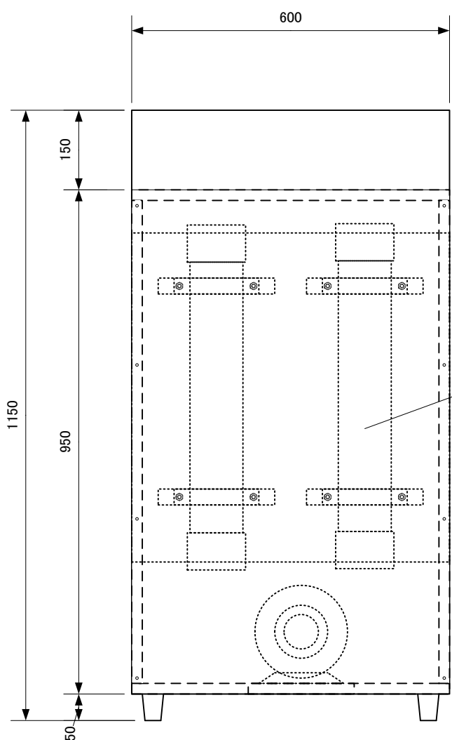
【背面】
